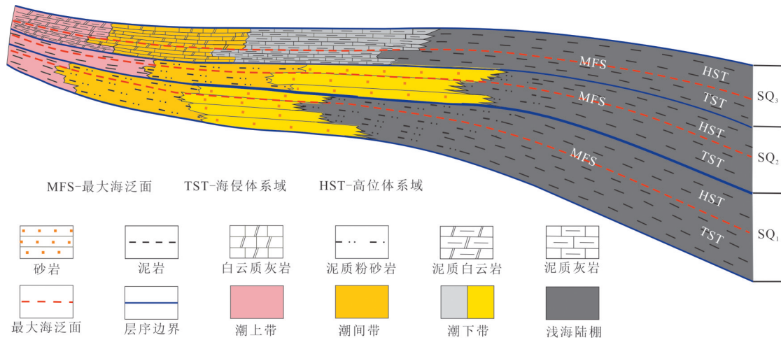
图8 华北龙山地区青白口系层序地层发育模式
