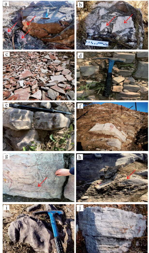
图5 华北龙山地区景儿峪组岩性特征
