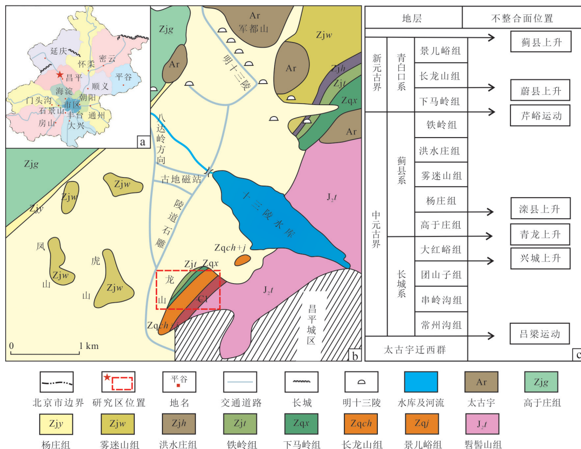
图1 华北龙山地区位置图及中、新元古界发育特征
